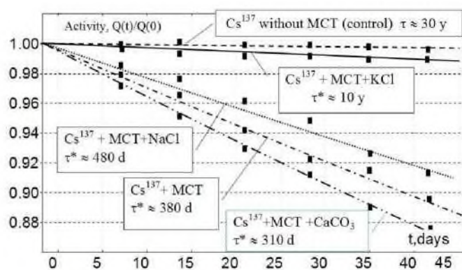
Рис. 8. Результаты экспериментов по трансмутации реакторного изотопа Cs^{137} .
