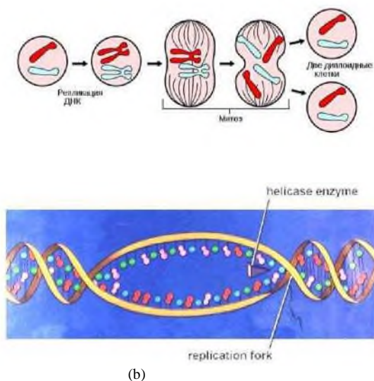
Рис. 10. Примеры формирования нестационарных потенциальных ям в биологических макромолекулах в пространстве между разделяющимися клетками (а) и в области расщивания ДНК в процессе репликации (б), в пределах которых реализуются условия формирования когерентных коррелированных состояний.
