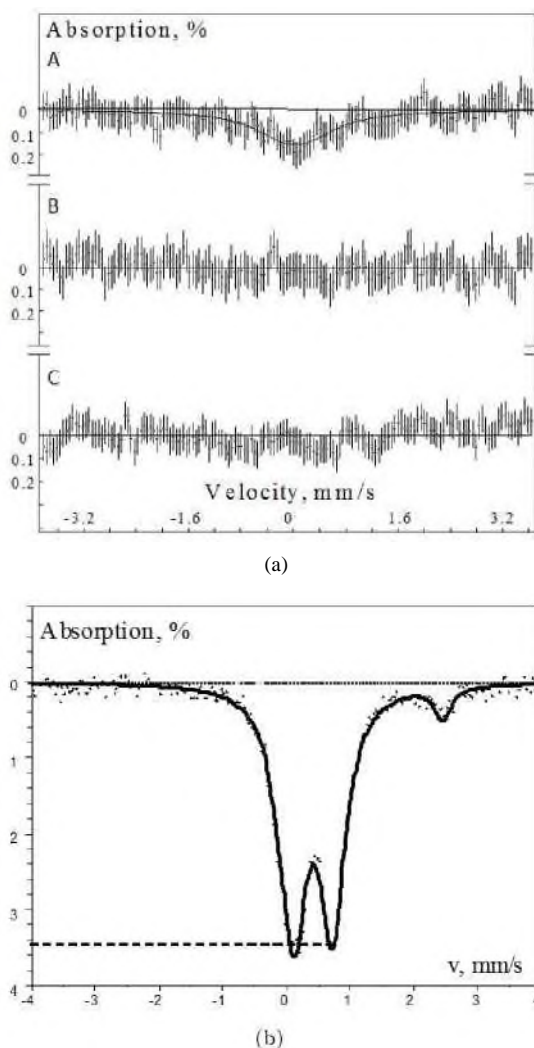
Рис. 1. а) Мессбауэровский спектр высушенной культуры Saccharomyces cerevisiae , выросшей в среде, содержащей: А - D2O и изотоп \text{Mn}^{55} ; В - \text{H}_2\text{O} и тот же изотоп \text{Mn}^{55} ; С - D2O без наличия \text{Mn}^{55} . б) мессбауэровский спектр высушенной синтрофной микробиологической ассоциации, выросшей в оптимальной среде при наличии D2O и изотопа \text{Mn}^{55} .
