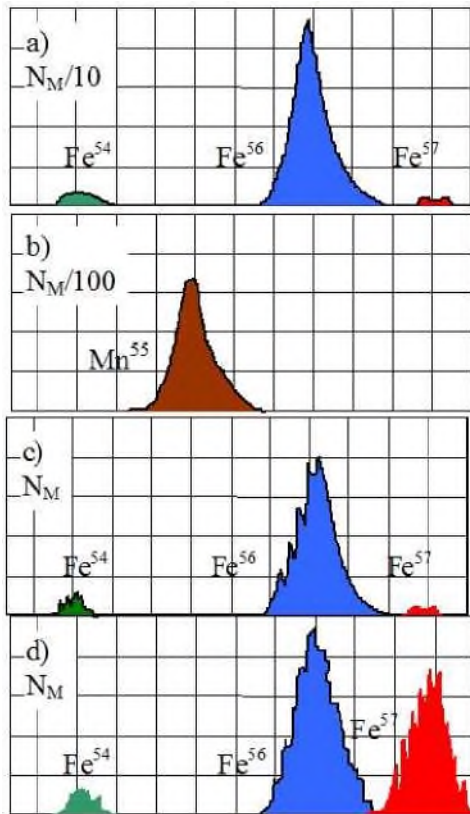
Рис. 3. Результаты измерения спектра изотопов в интервале массовых чисел A=[54...57] для а) — природного железа; б) чистого марганца; в) отмытой и высушенной культуры, выросшей в контрольной среде на основе легкой воды с присутствием марганца; д) отмытой и высушенной культуры, выросшей в среде на основе тяжелой воды, содержащей соли марганца.
