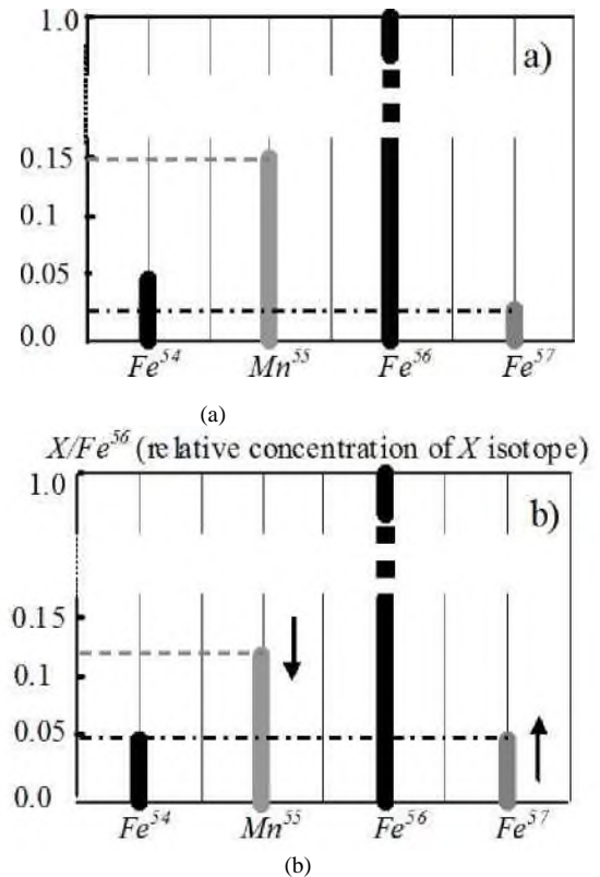
Рис. 5. Спектр масс в области A=54-57 высушенной микробиологической ассоциации, выросшей в контрольной среде на основе легкой воды H_2O при наличии изотопа Mn^{55} и исследованной совместно с сухими компонентами питательной среды (a) и в оптимальной среде на основе тяжелой воды D_2O в присутствии того же изотопа Mn^{55} (b).
