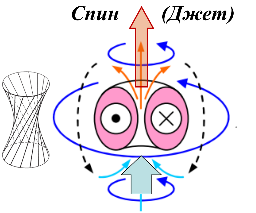
Эфиродинамическая схема протона, атома, кавитац. пузырька, ... , галактик
