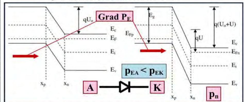
p-n переход при обратном смещении U_0 .
