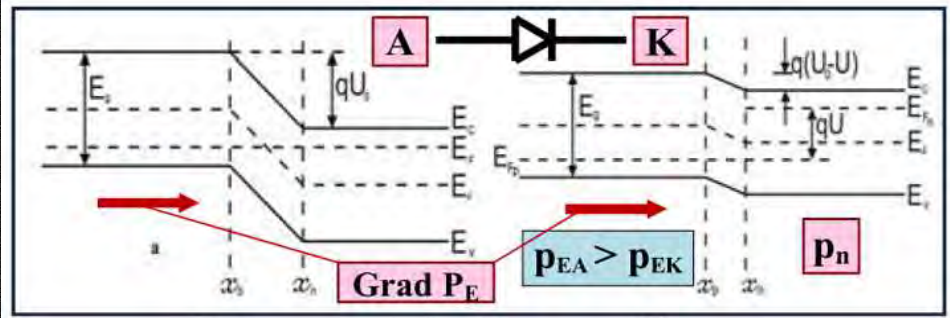
p-n переход при прямом смещении U_0 .
