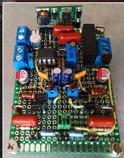
Усилитель – Формирователь
