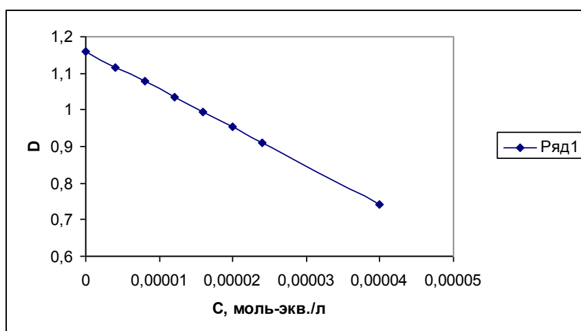
Рисунок 2. Зависимость оптической плотности раствора K_3[Fe(CN)_6]/K_4[Fe(CN)_6] (начальная концентрация K_3[Fe(CN)_6]=2,24 \times 10^{-4} ) от концентрации гидрохинона. l=5 см
