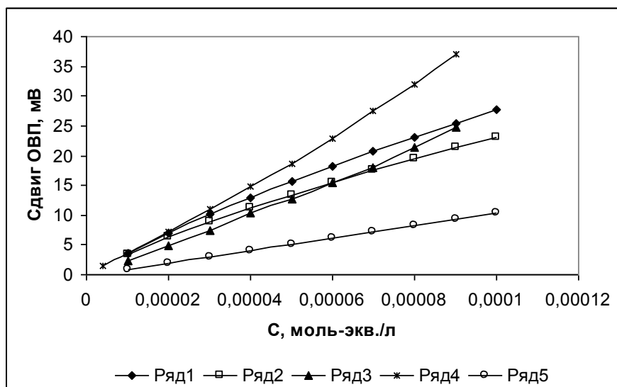
Рисунок 1. Зависимость сдвига ОВП от концентрации аскорбиновой кислоты для медиаторных систем K_4[Fe(CN)_6]/K_3[Fe(CN)_6] : 1- 5 \times 10^{-5}/2 \times 10^{-4} M ; 2 - 5 \times 10^{-5}/5 \times 10^{-4} M ; 3 - 2 \times 10^{-4}/2 \times 10^{-4} M ; 4 - 7,5 \times 10^{-5}/7,5 \times 10^{-5} M ; 5 - 5 \times 10^{-4}/5 \times 10^{-4} M ;
