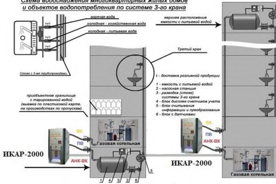
Схема водоснабжения многоквартирных жилых домов и объектов водопотребления по системе 3-го крана
